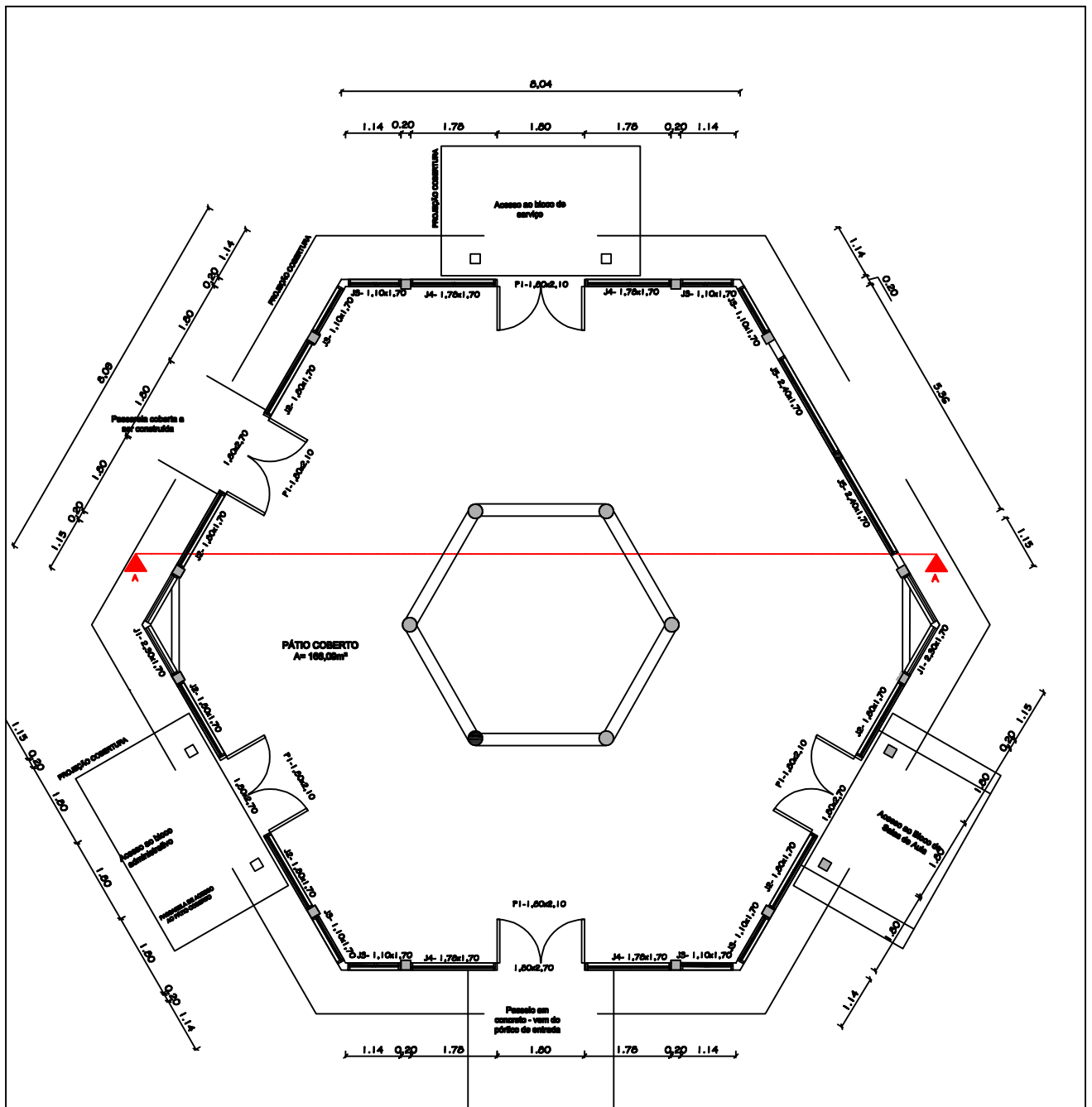
Planta Baixa do Fechamento do Pátio Coberto Escala 1:125 Área 175,35m 2
