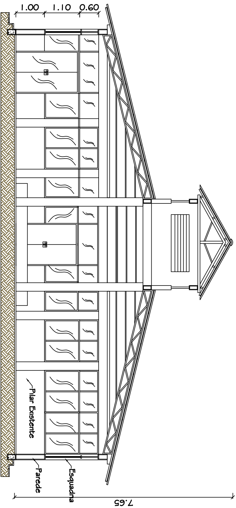
Corte A-A Escala 1:75
