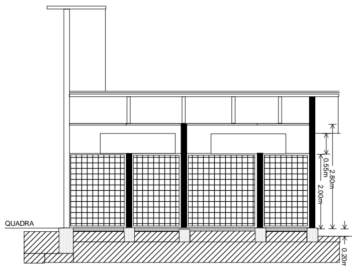
CORTE
